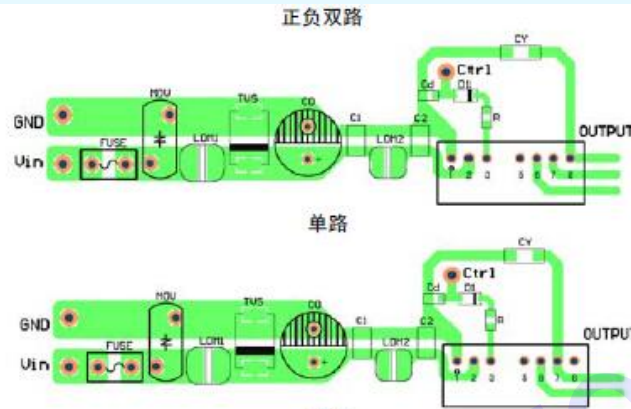
图 2 注：输入输出地之间(CY)焊盘最小距离要保证≥2mm。
